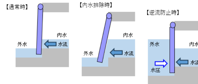
フラップゲートの仕組み
